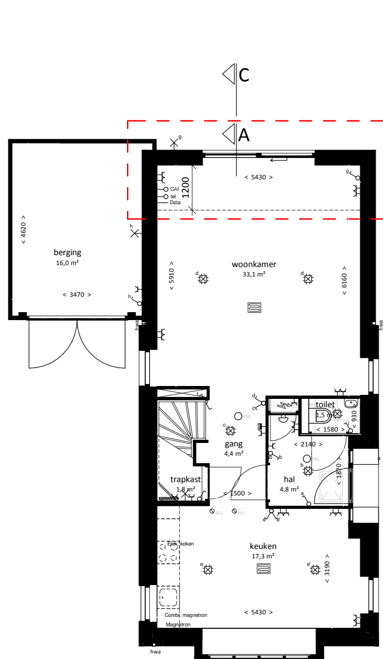
Begane grond uitbouw 1,2m in de achtergevel
