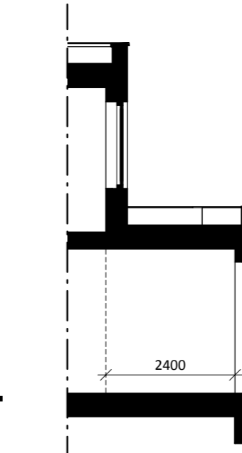
Doorsnede B 2,4m uitbouw in de achtergevel op de begane grond
