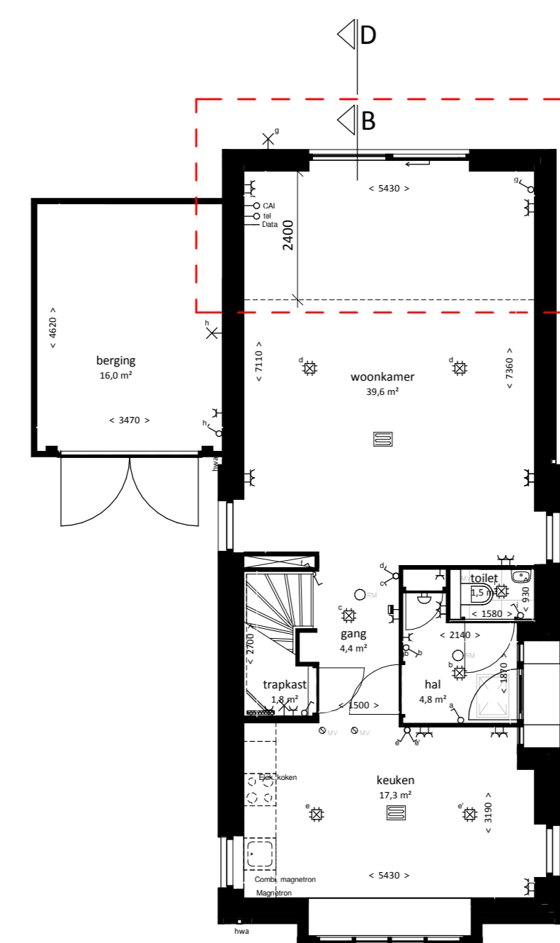
Begane grond uitbouw 2,4m in de achtergevel
