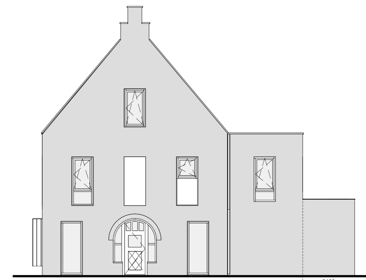
Zijgevel rechts uitbouw 2,4m op de begane grond
