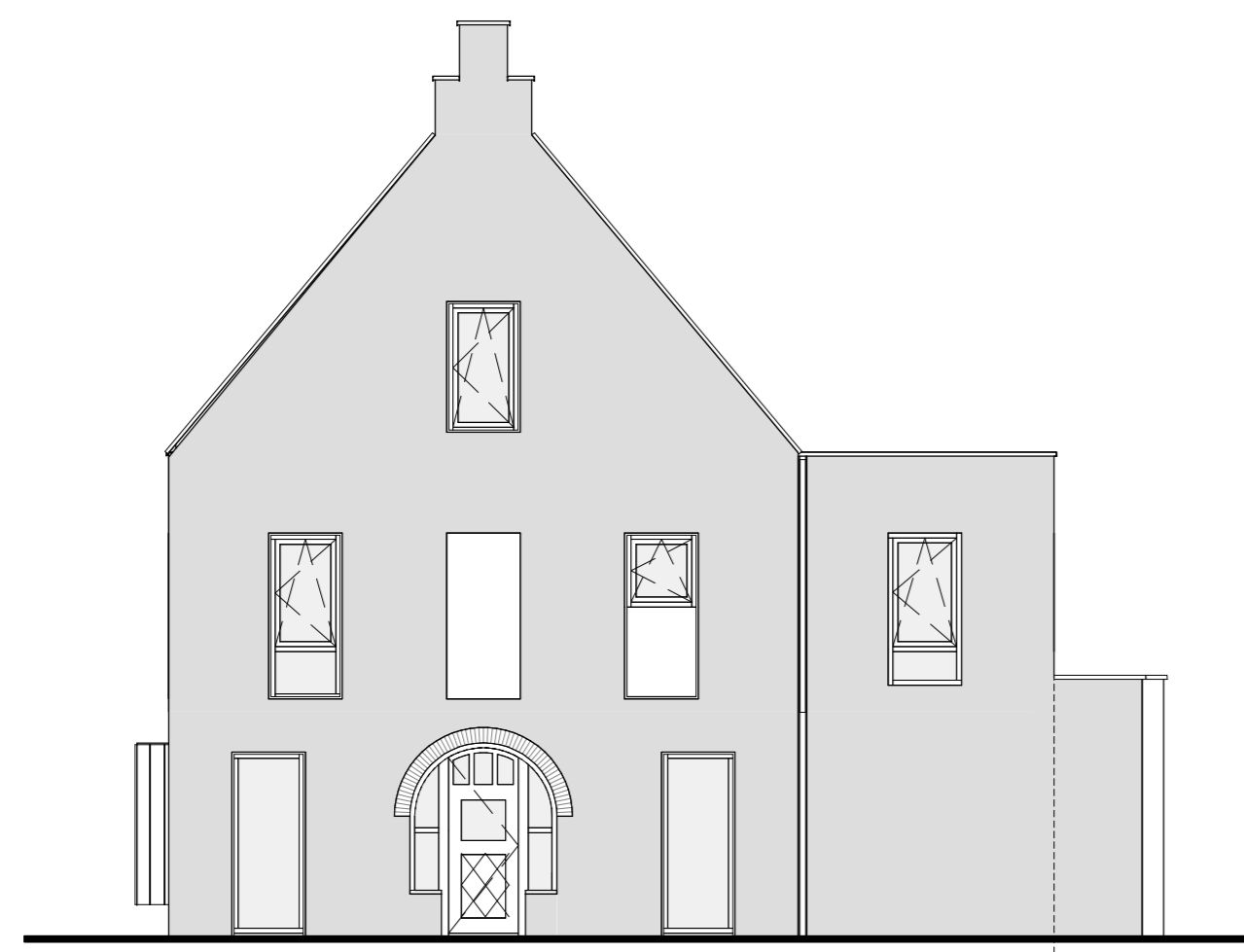
Zijgevel rechts uitbouw 1,2m op de begane grond
