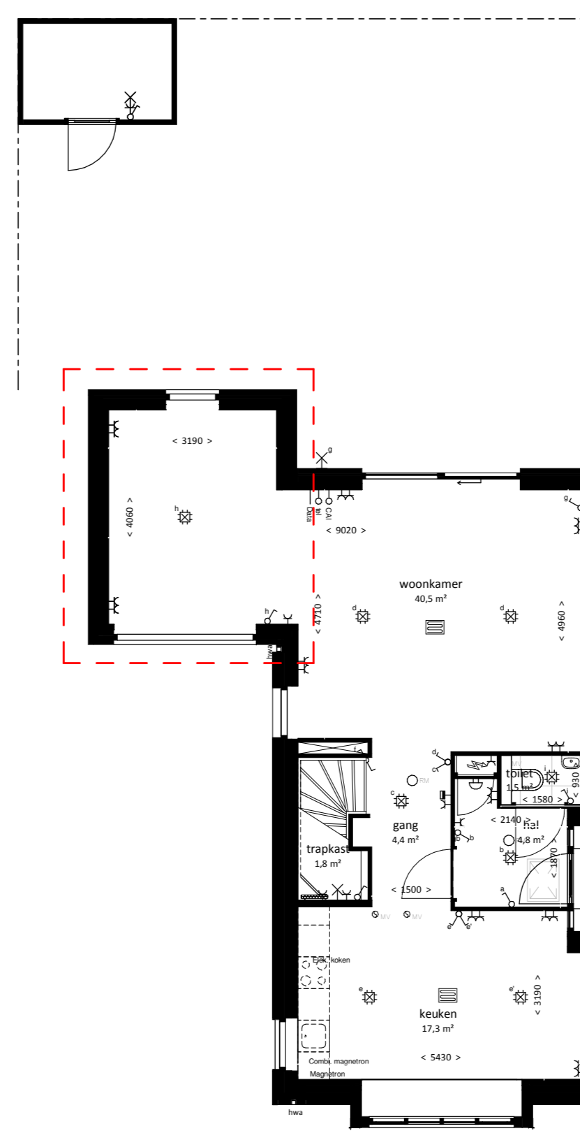
Begane grond berging bij woonkamer
