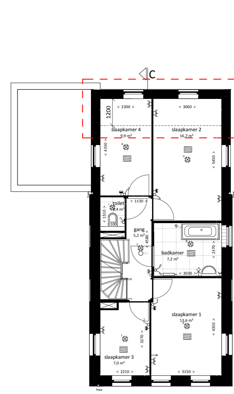
1e verdieping uitbouw 1,2m in de achtergevel
