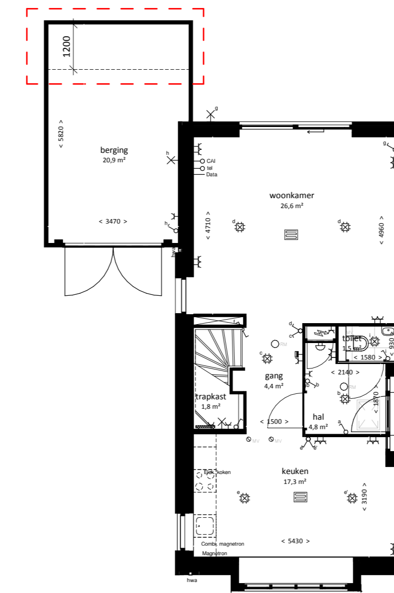
Begane grond uitbouw berging 1,2m
