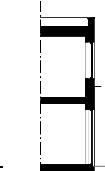
Doorsnede C 1,2m uitbouw in de achtergevel op de begane grond en 1e verdieping
