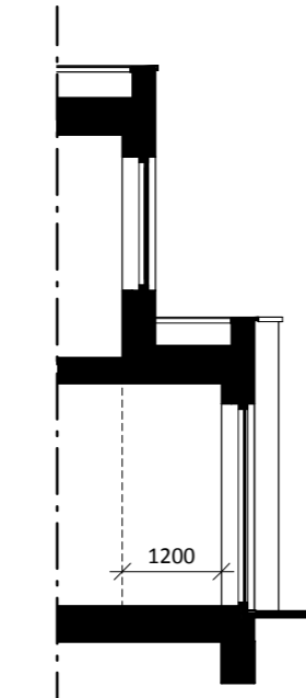
Doorsnede A 1,2m uitbouw in de achtergevel op de begane grond
