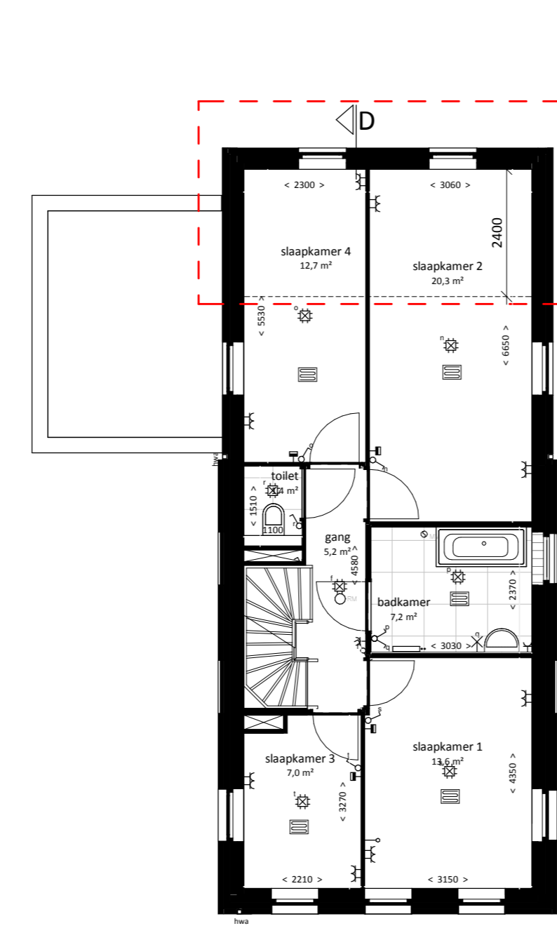
1e verdieping uitbouw 2,4m in de achtergevel
