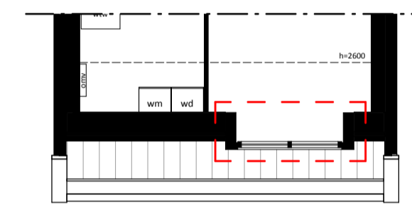
Verdieping 02
