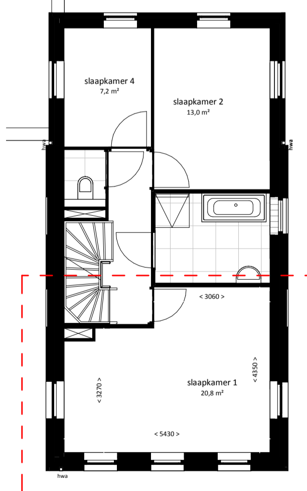
Verdieping 01 optie 12a
