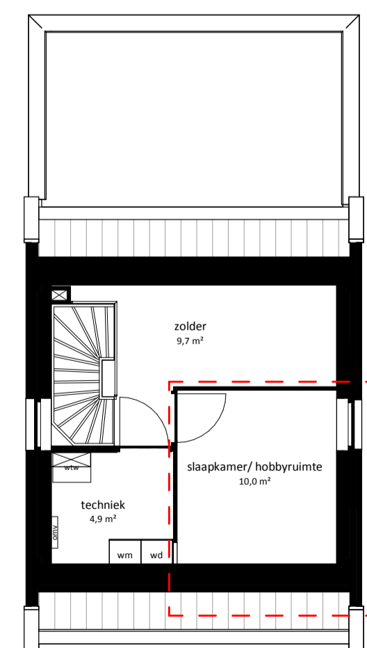
Verdieping 02 Optie 13a
