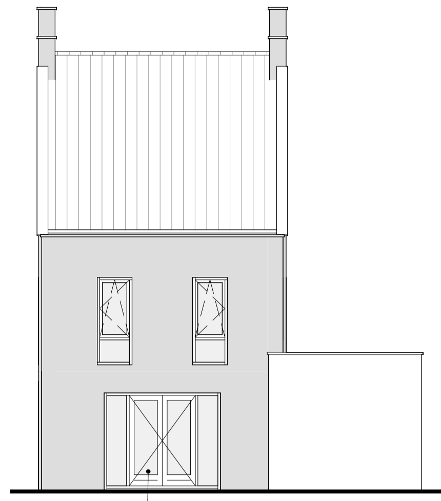
loopdeur Achtergevel
