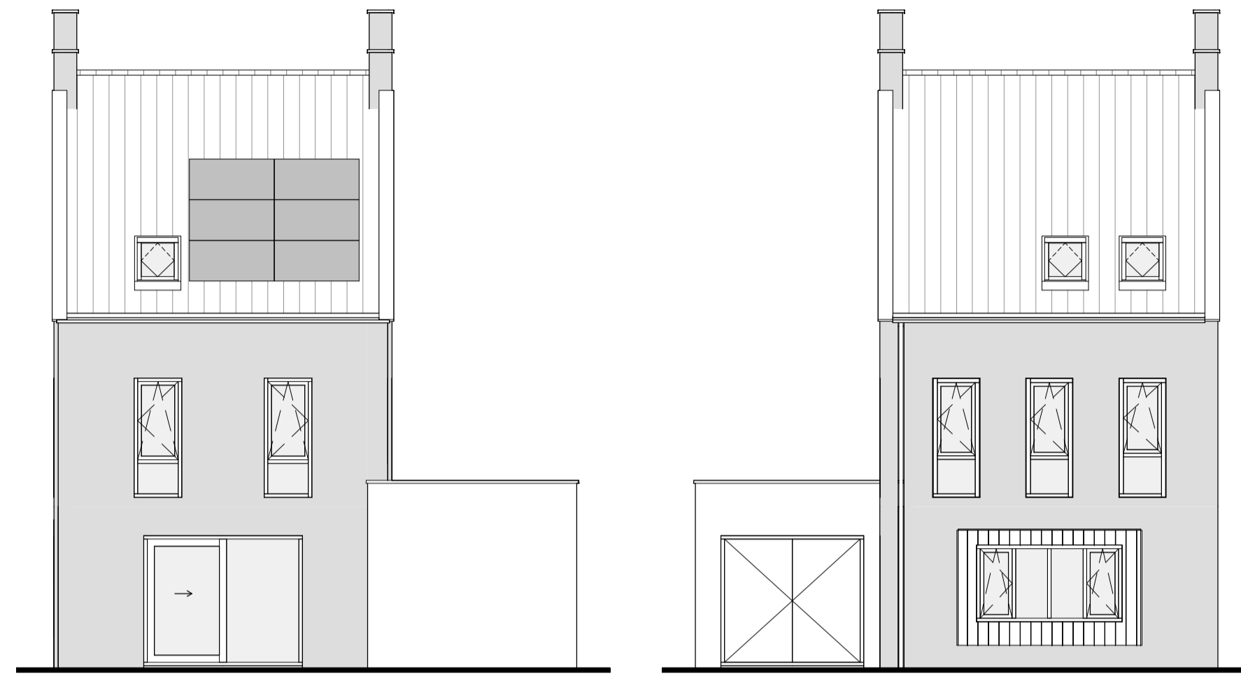
Achtergevel
