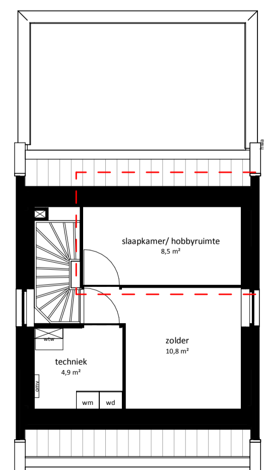
Verdieping 02 Optie 13b
