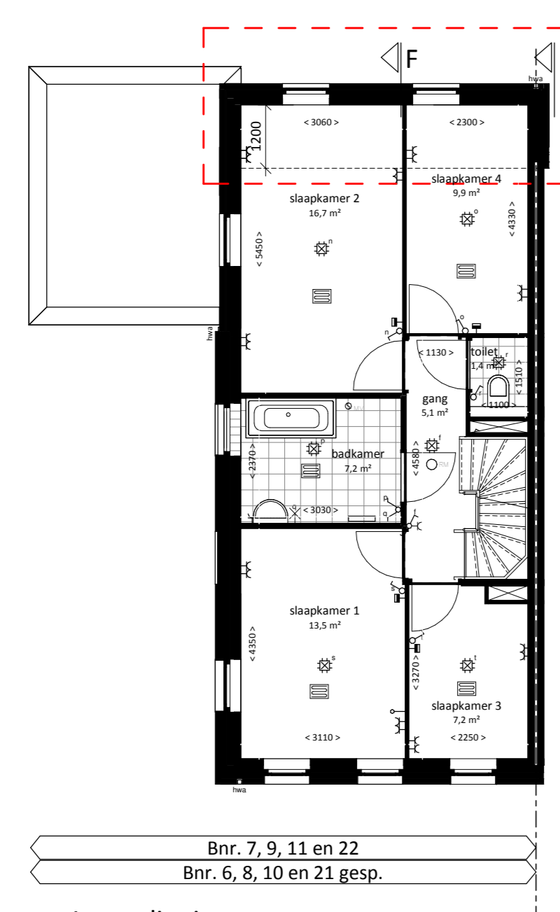
1e verdieping uitbouw 1,2m in de achtergevel
