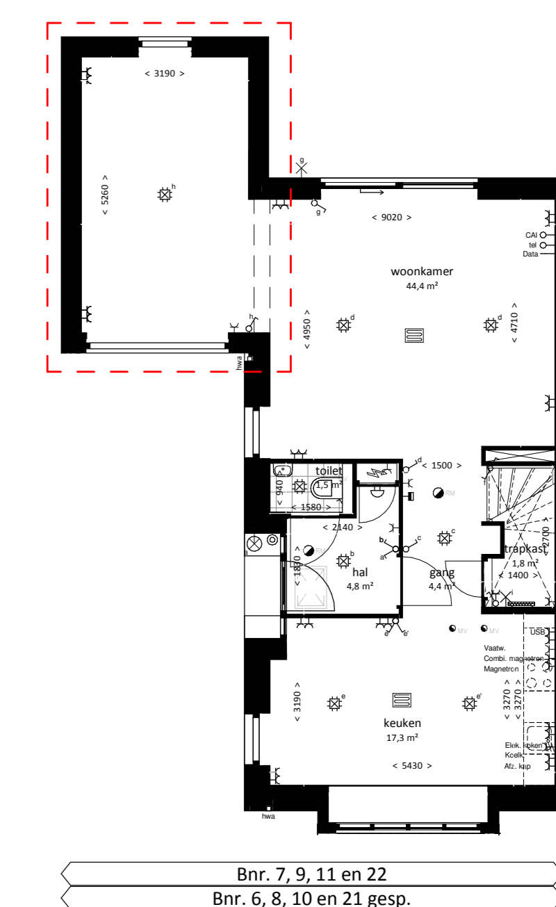
Begane grond uitbouw berging bij woonkamer
