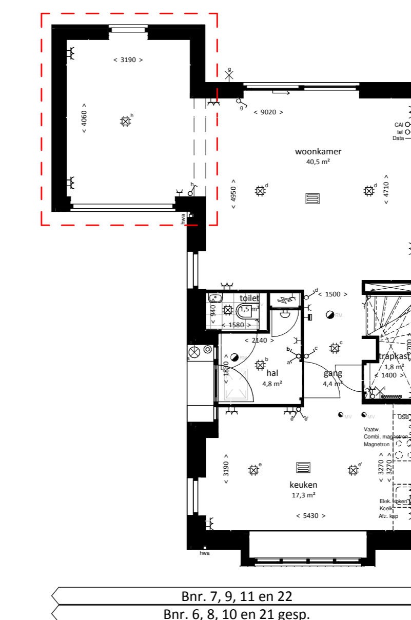
Begane grond berging bij woonkamer
