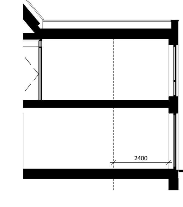
Doorsnede G uitbouw 2,4m in de achtergevel
