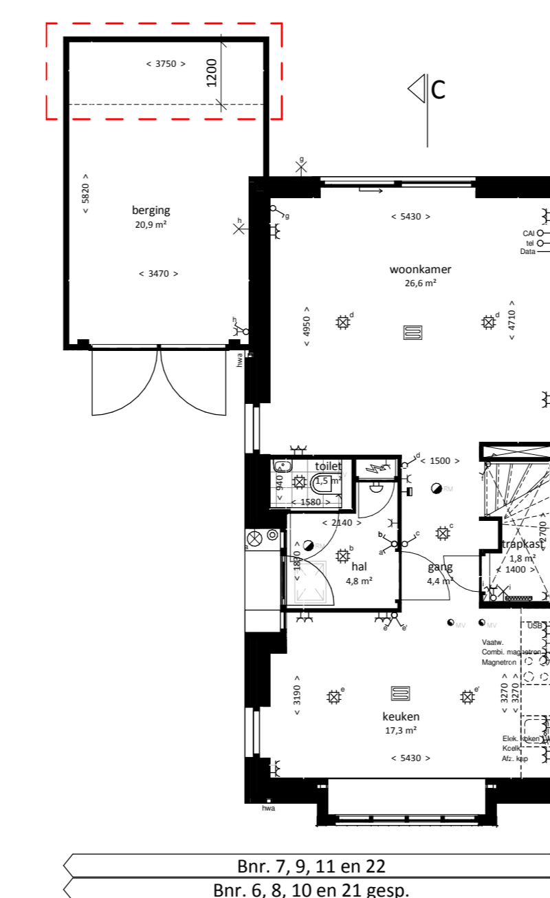
Begane grond uitbouw berging 1,2m
