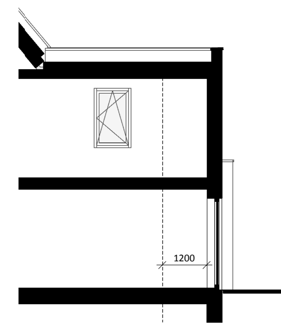
Doorsnede F uitbouw 2,4m in de achtergevel
