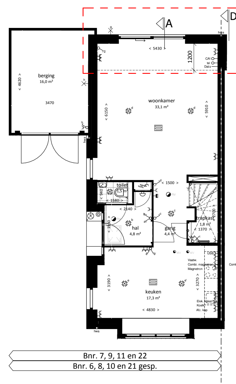
Begane grond uitbouw 1,2m in de achtergevel
