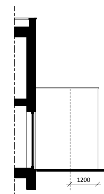
Doorsnede C uitbouw berging 1,2m
