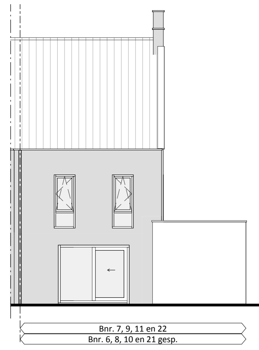
Achtergevel uitbouw 1,2m op de begane grond en verdieping
