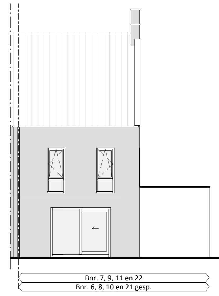
Achtergevel uitbouw 2,4m op de begane grond en verdieping
