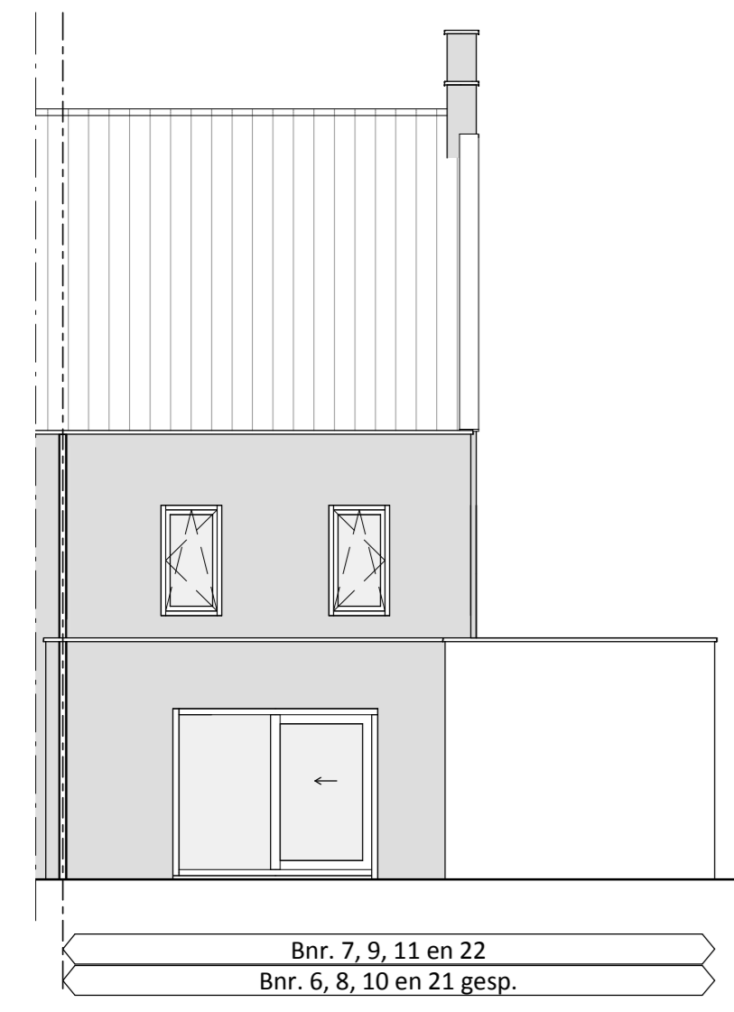
Achtergevel uitbouw 1,2m op de begane grond
