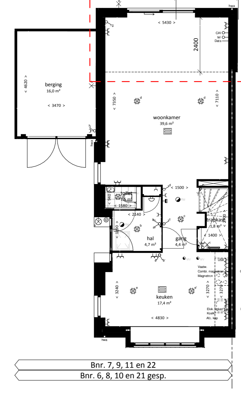
Begane grond uitbouw 2,4m in de achtergevel
