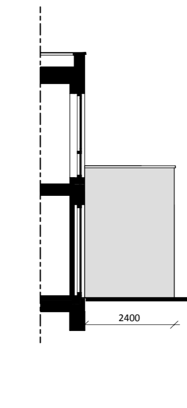
Doorsnede E uitbouw 2,4m in de achtergevel
