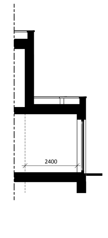
Doorsnede B uitbouw 2,4m in de achtergevel
