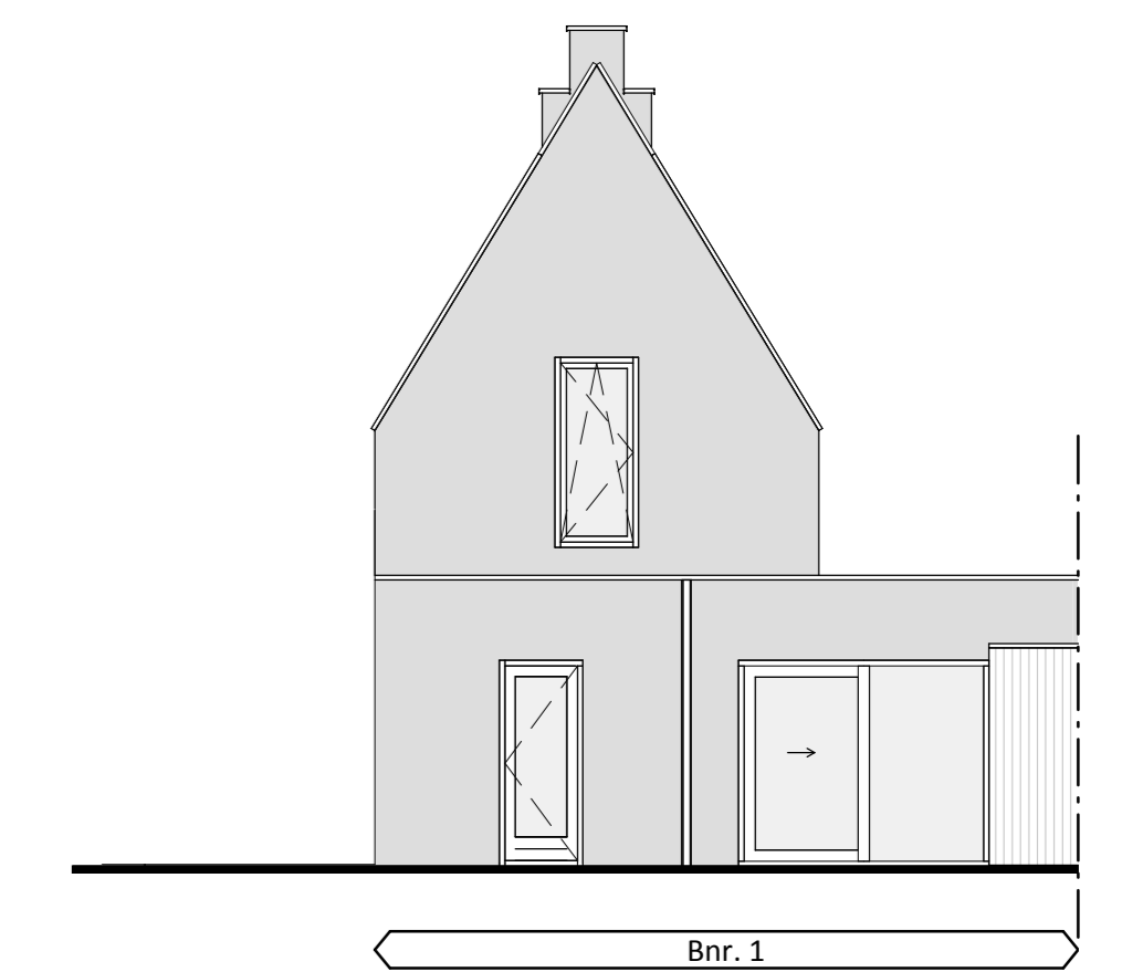
Achtergevel Bnr. 1 slaapkamer 1 begane grond ipv raam een deur
