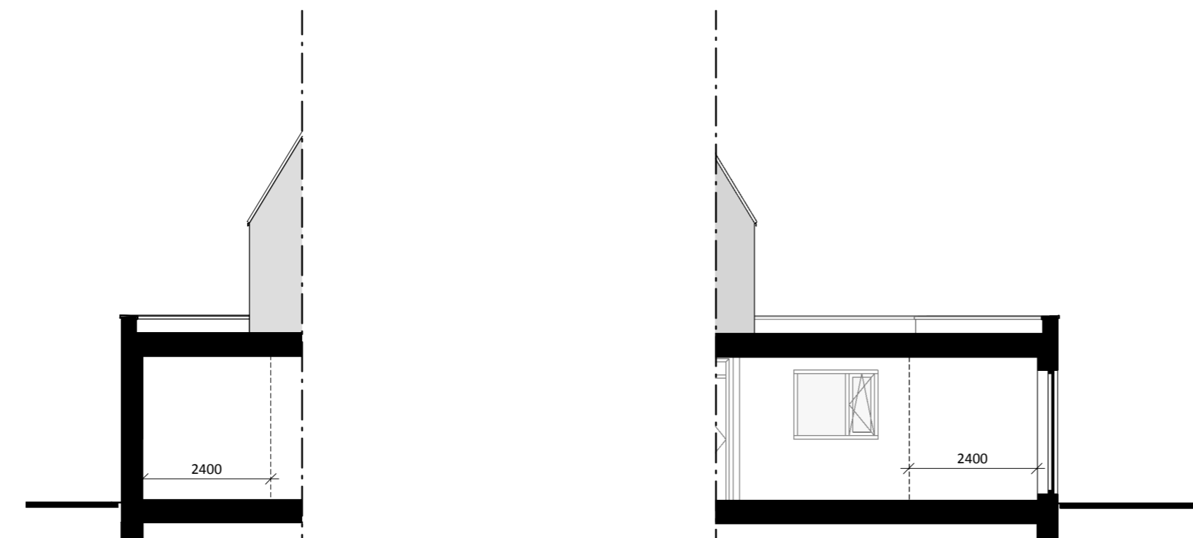
Doorsnede C uitbouw 2,4m Bnr. 1
