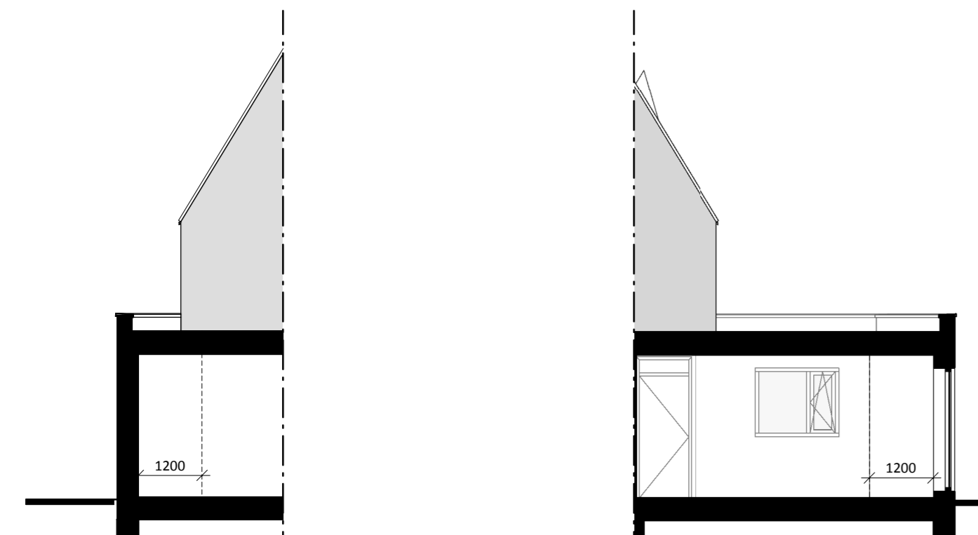
Doorsnede A uitbouw 1,2m Bnr. 1
