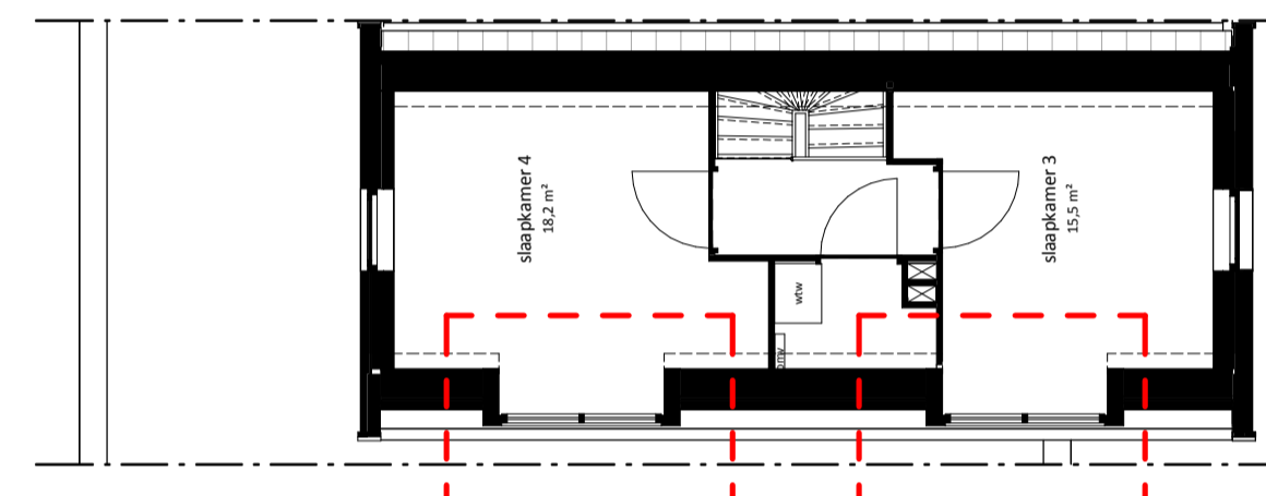
Verdieping 01 optie 7a dakkapel 2m breed
