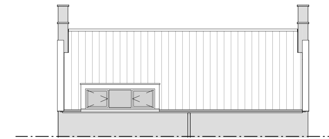
Zijgevel optie 7b dakkapel 3m breed
