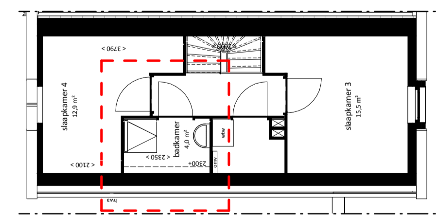
Verdieping 01 optie extra badkamer
