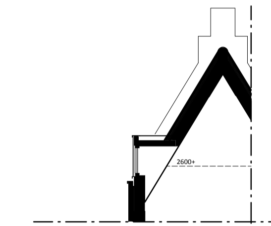
Doorsnede
