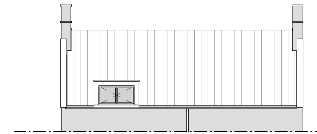
Zijgevel optie 7a dakkapel 2m breed
